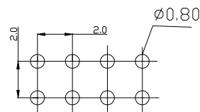
P.C.B Hole Layout
