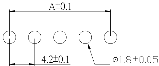
P.C.B. hole dimensions
